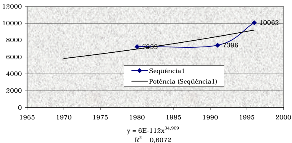
Curva Potência de Crescimento - Ararendá
