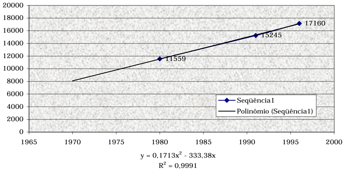
Curva Polinomial de Crescimento - Forquilha
