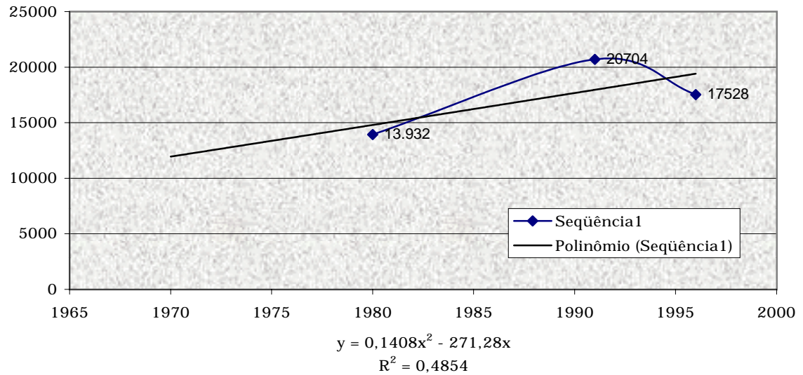
Curva Polinomial de Crescimento - Marco
