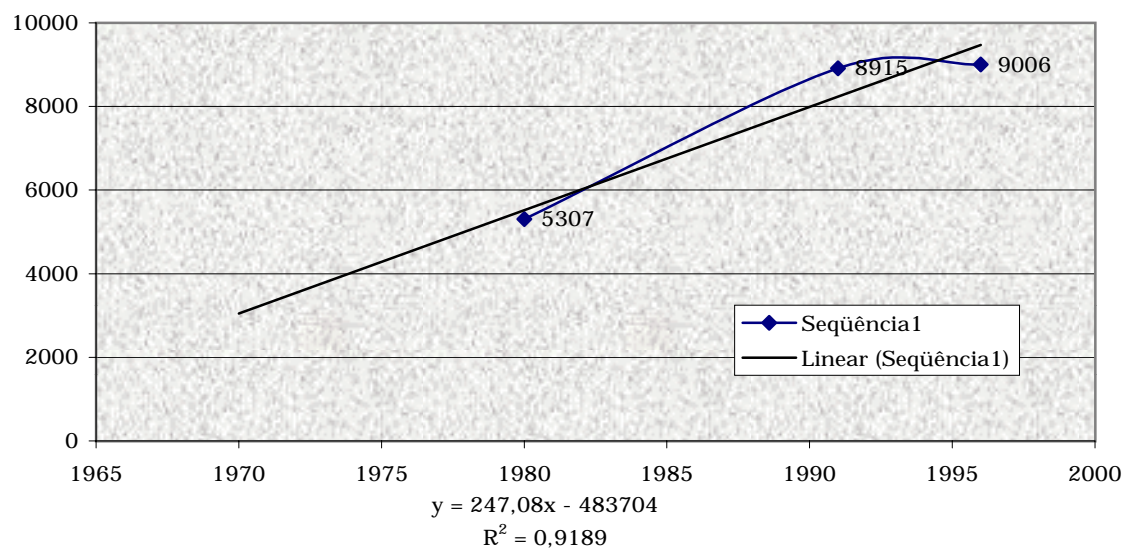
Curva Linear de Crescimento - Catunda
