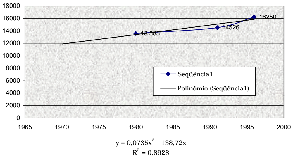
Curva Polinomial de Crescimento - Morrinhos
