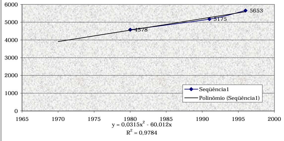
Curva Polinomial de Crescimento - Senador Sá
