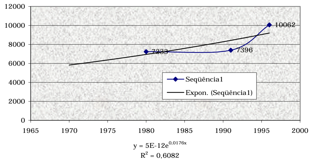
Curva Exponencial de Crescimento - Ararendá
