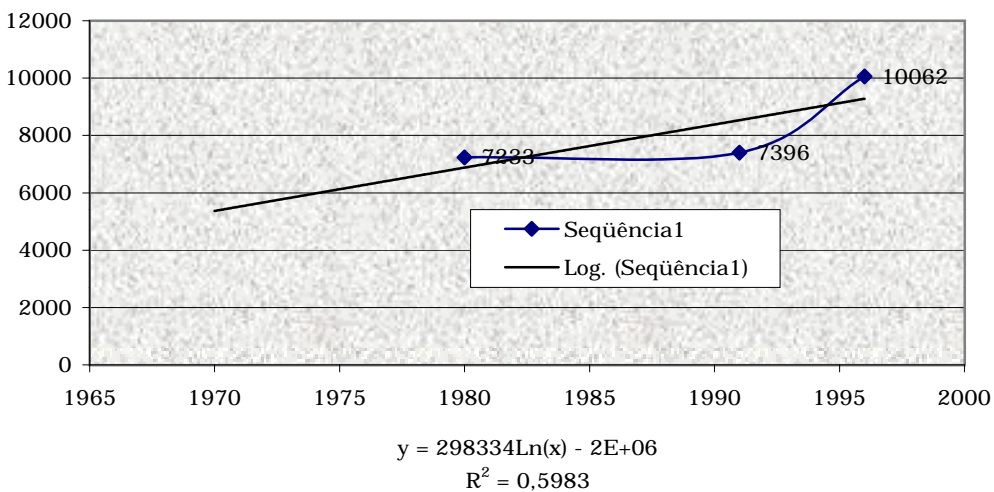
Curva Logarítmica de Crescimento - Ararendá
