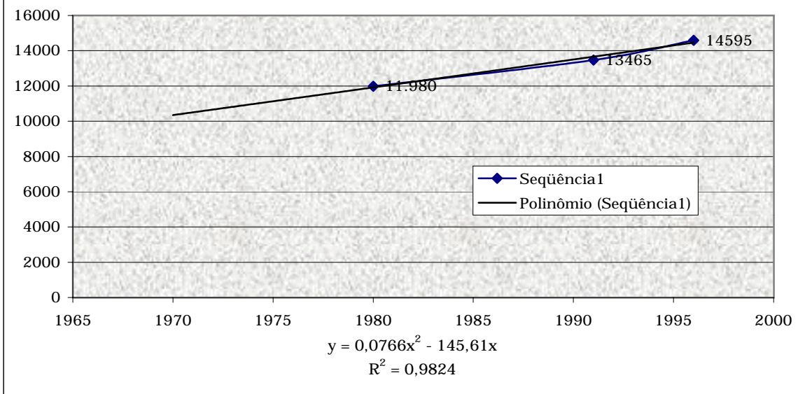
Curva Polinomial de Crescimento - Varjota
