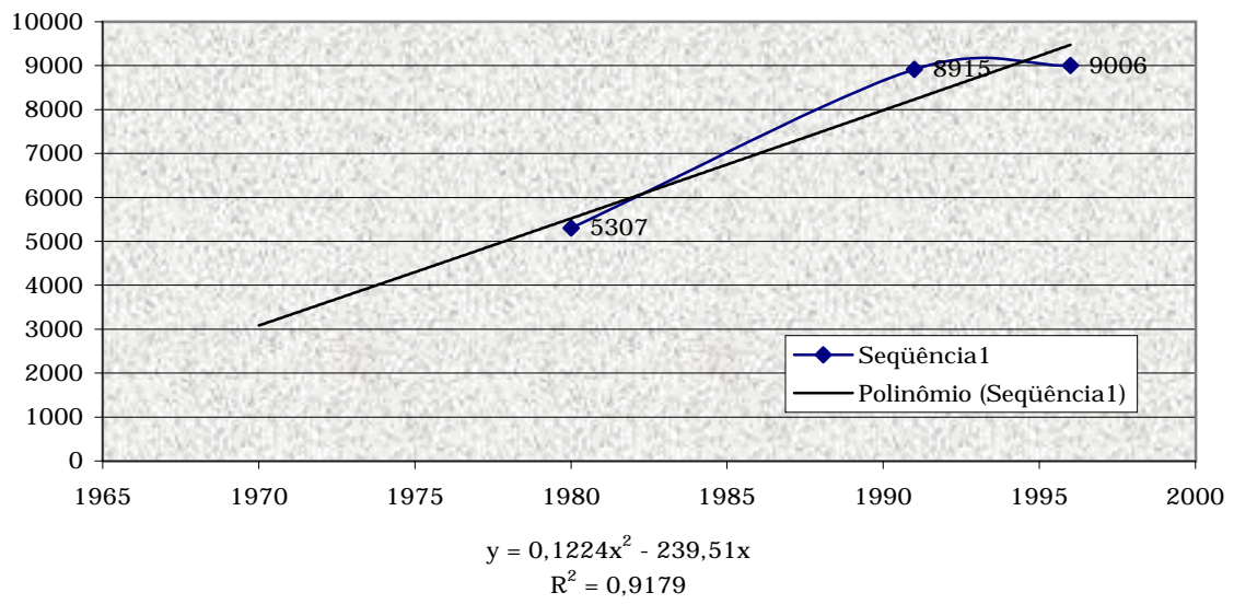
Curva Polinomial de Crescimento - Catunda
