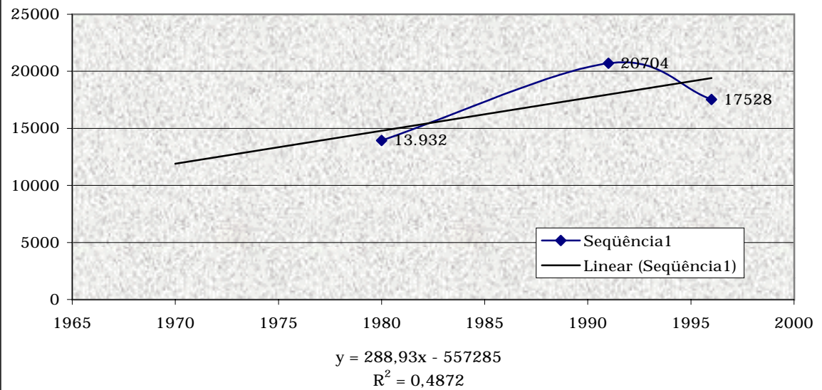
Curva Linear de Crescimento - Marco
