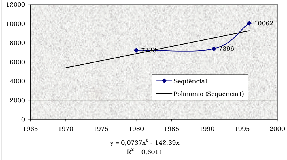
Curva Polinomial de Crescimento - Ararendá
