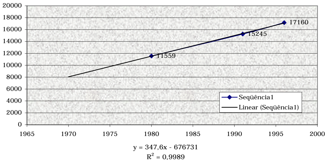
Curva Linear de Crescimento - Forquilha
