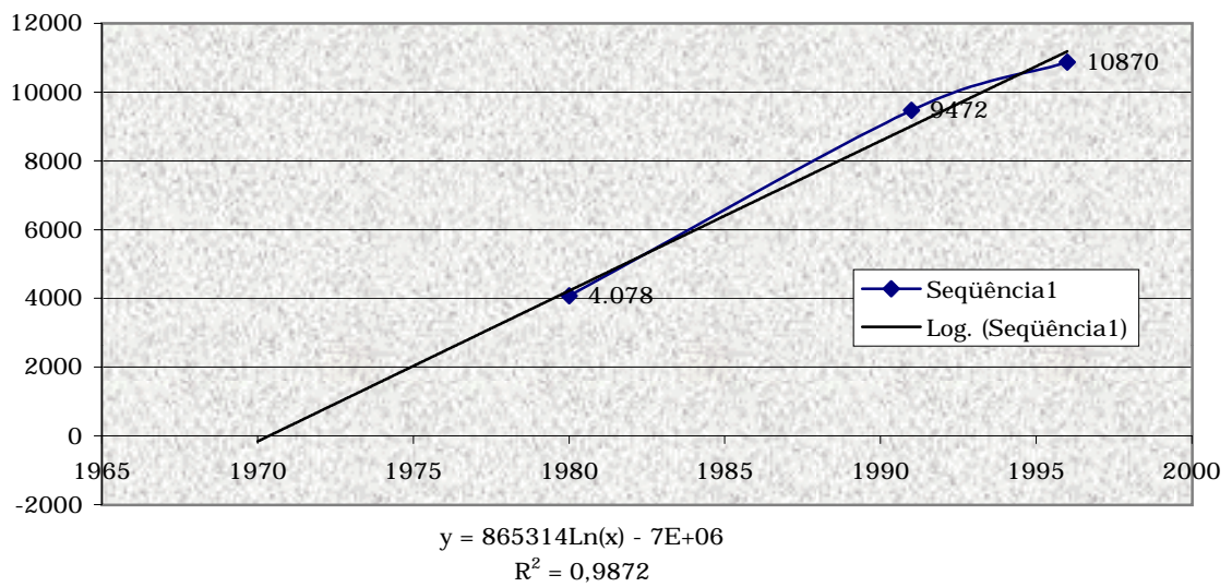
Curva Logarítmica de Crescimento - Pires Ferreira
