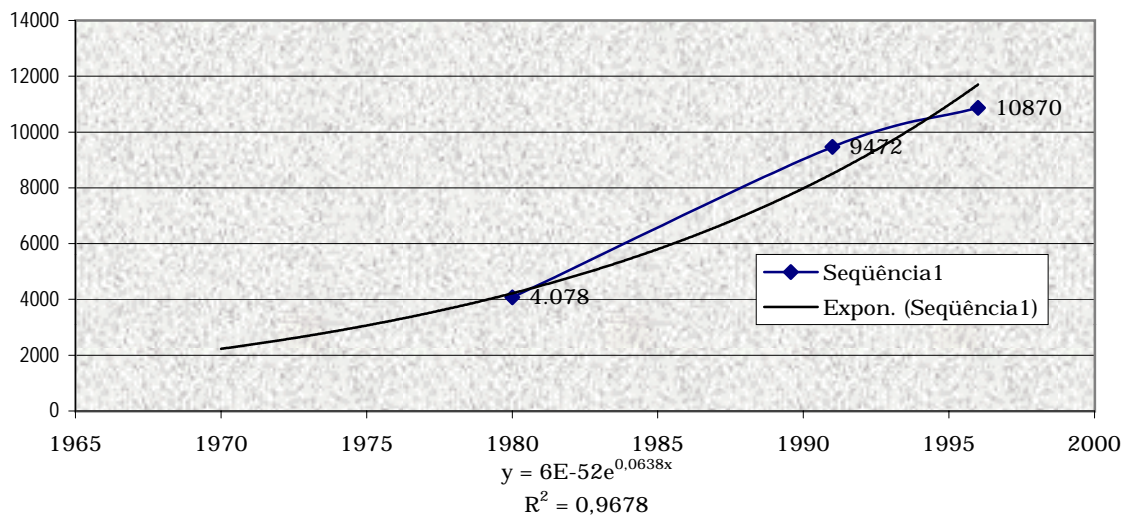
Curva Exponencial de Crescimento - Pires Ferreira
