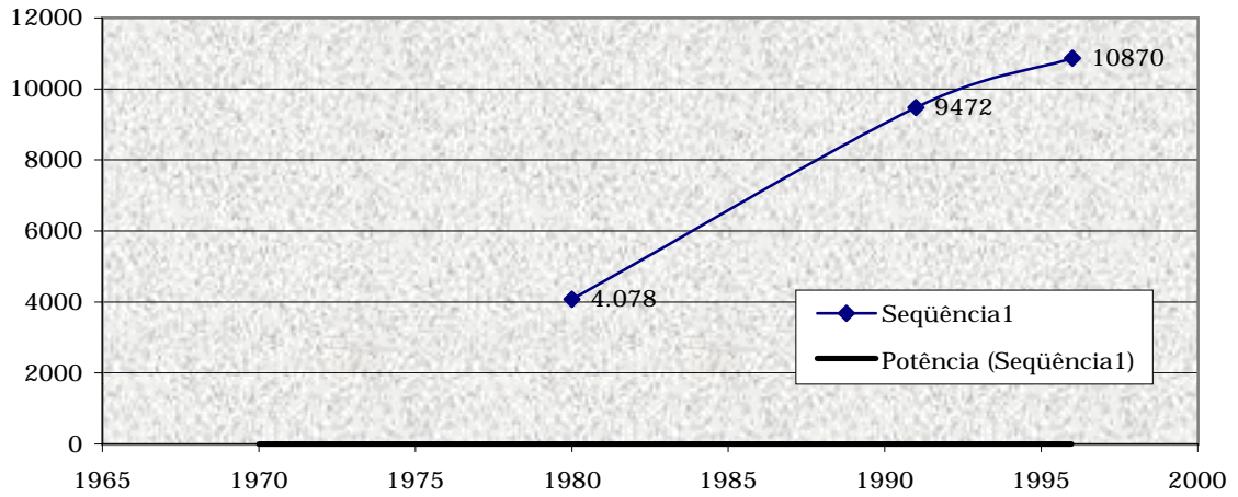
Curva Potência de Crescimento - Pires Ferreira
