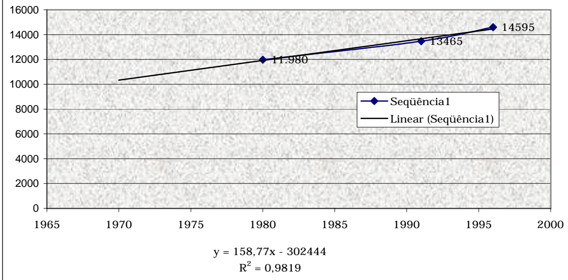
Curva Linear de Crescimento - Varjota
